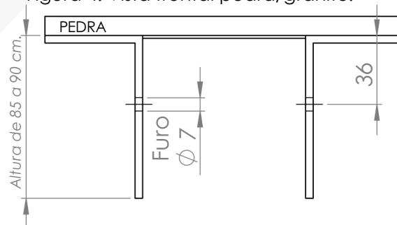
Figura 4: Vista frontal pedra/granito.
