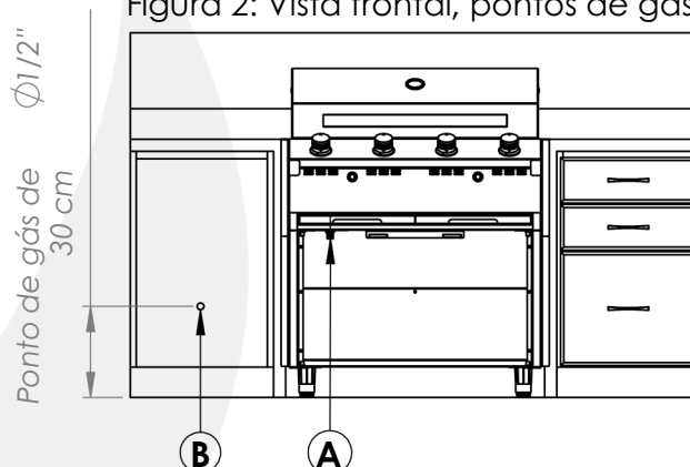
Figura 2: Vista frontal, pontos de gás.
