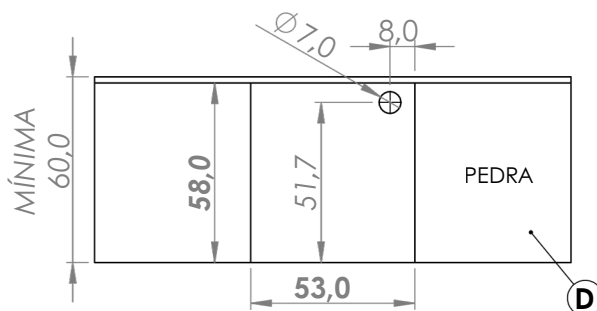
Figura 3: Vista superior pedra/granito.
