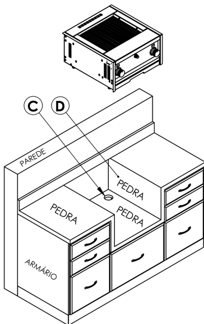
Figura 1: Vista isométrica.
