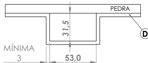
Figura 4: Vista frontal pedra/granito.
