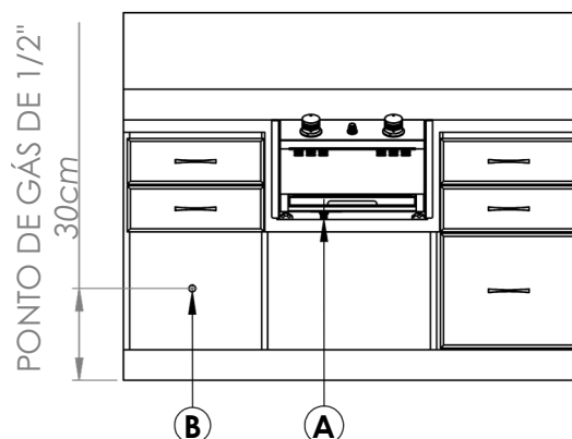
Figura 2: Vista frontal, pontos de gás.
