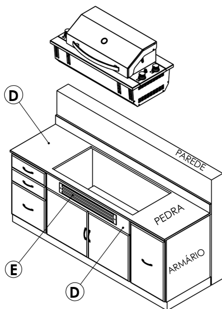
Figura 1: Vista isométrica.
