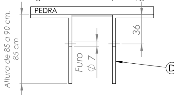
Figura 4: Vista frontal pedra/granito.
