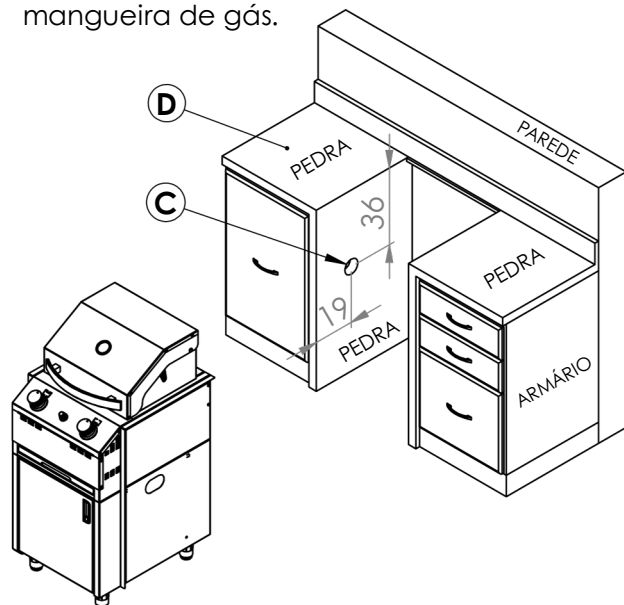
Figura 1: Furo na pedra para passagem de mangueira de gás.
