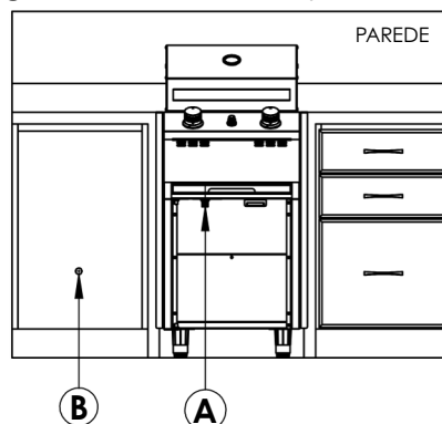
Figura 2: Vista frontal, pontos de gás.
