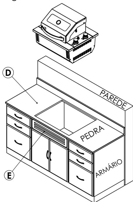
Figura 1: Vista isométrica.
